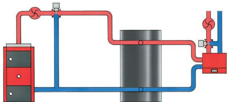
Holzfeuerungskessel mit integrierter Speicherladung
