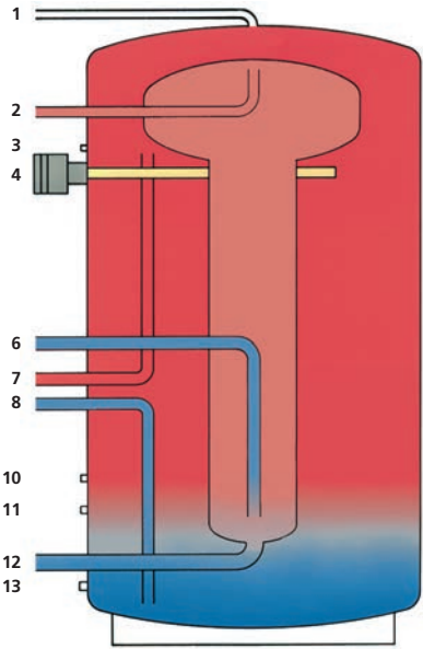
Für reine Holzfeuerung
